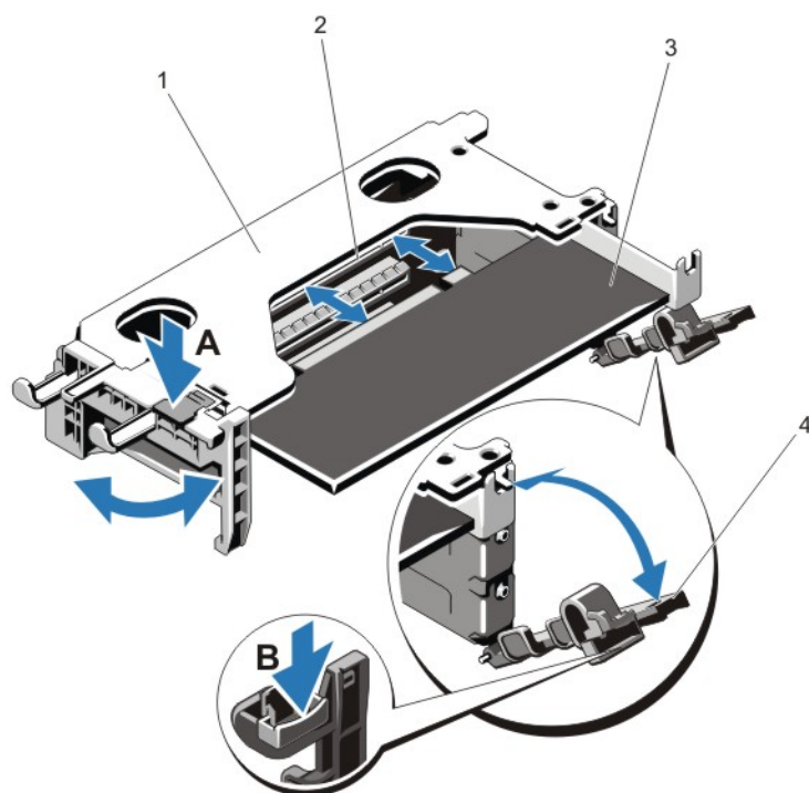
図 25. 拡張カードライザー 1 の取り外しと取り付け
