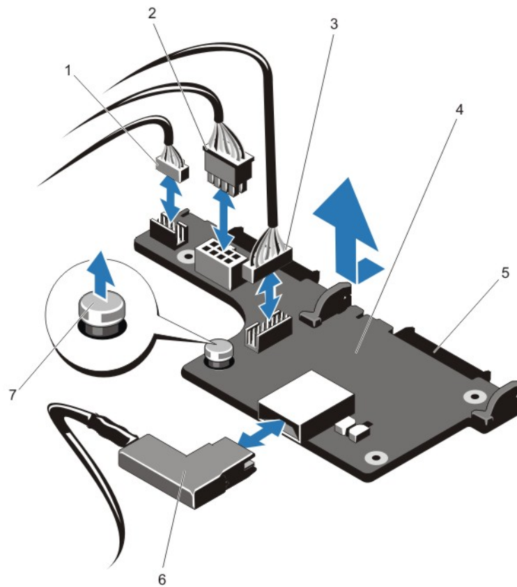
図 42. オプションの 2.5 インチ (x2) ハードドライブバックプレーンの取り外しと取り付け
