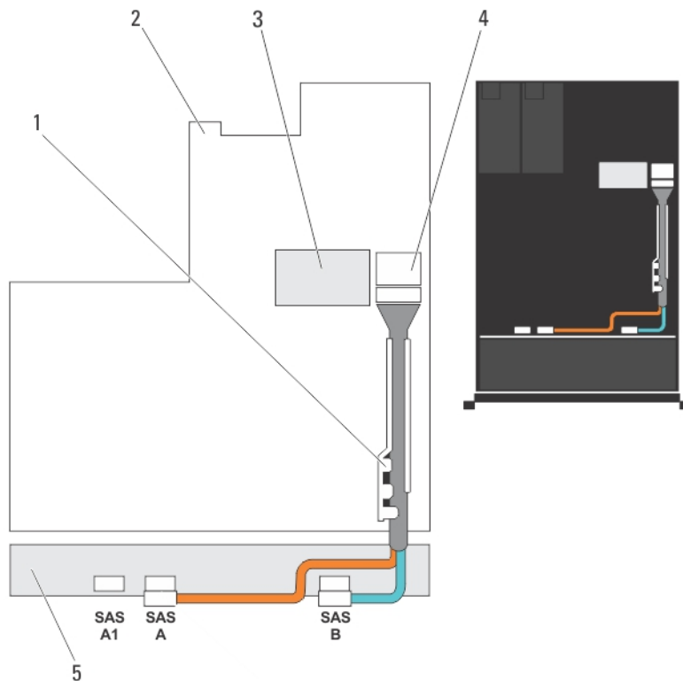
図 41. ケーブル接続図 – 3.5 インチ (x12) SAS バックプレーン
