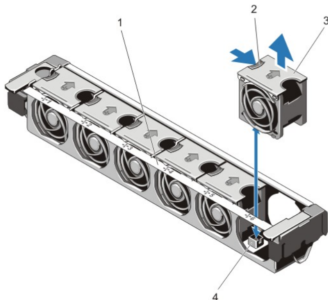
図 18. 冷却ファンの取り外しと取り付け
