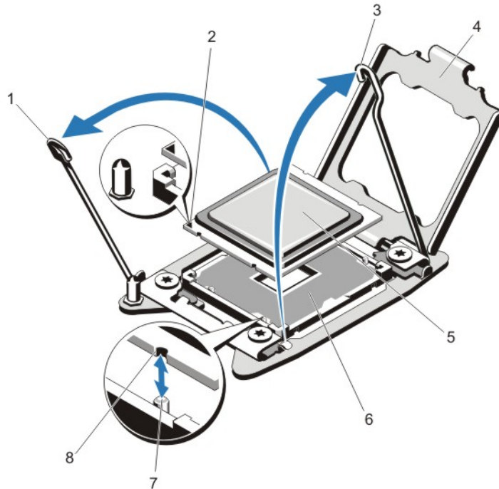
図 36. プロセッサの取り外しと取り付け
