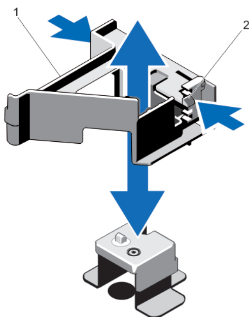
図 21. PCIe カードホルダの取り外しと取り付け
