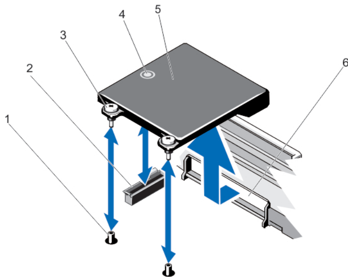
図 33. ネットワークドーターカードの取り外しと取り付け
