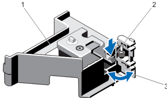
図 22. PCIe カードホルダラッチの開閉
