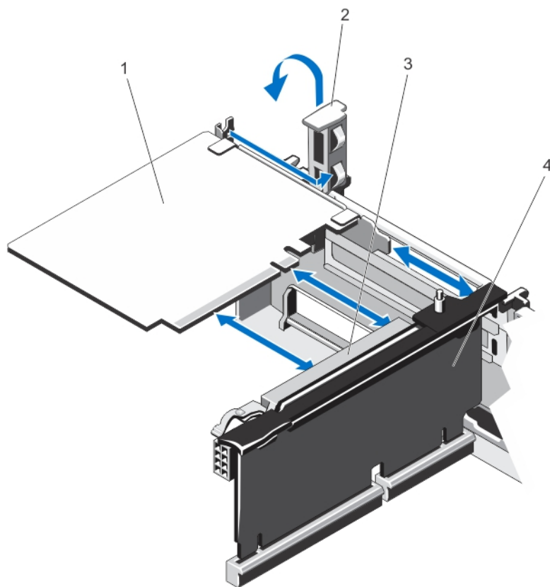
図 24. 拡張カードの取り外しと取り付け
