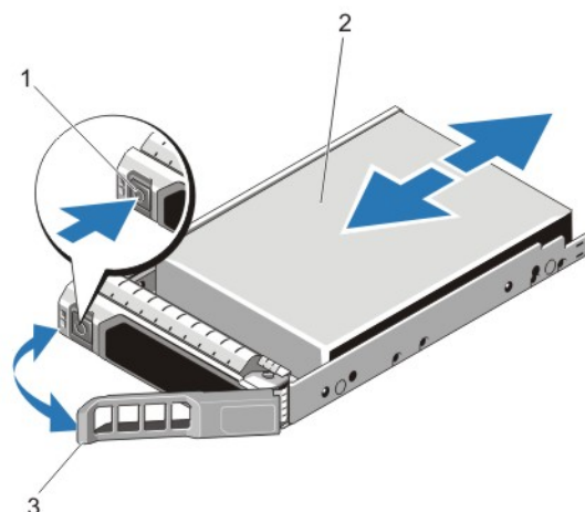
図 16. ホットスワップ対応ハードディスクドライブの取り外しと取り付け
