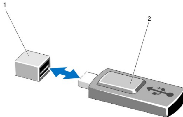
図 20. 内蔵 USB キーの交換
