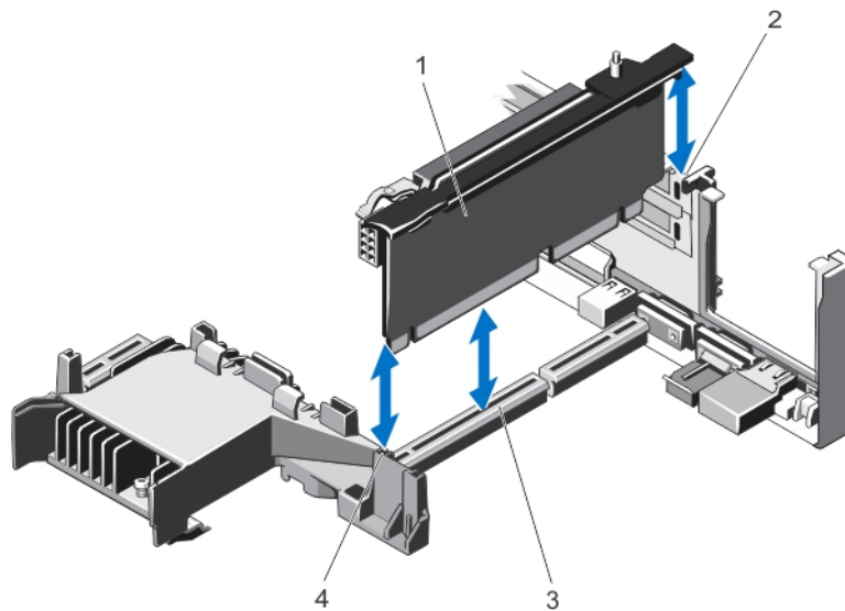
図 28. 拡張カードライザー 2 の取り外しと取り付け
