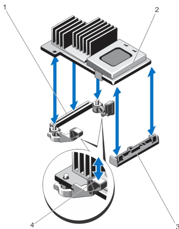
図 32. 内蔵ストレージコントローラカードの取り外しと取り付け
