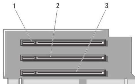
図 27. 拡張カードライザー 1 のコネクタの識別
