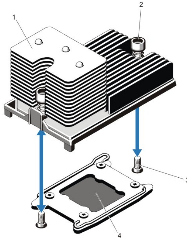
図 34. プロセッサヒートシンクの取り外しと取り付け
