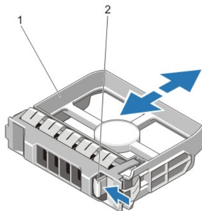
図 15. 3.5 インチハードドライブダミーの取り外しと取り付け
