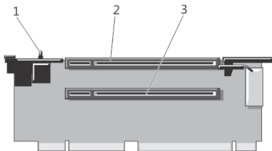
図 29. 拡張カードライザー 2 のコネクタの識別
