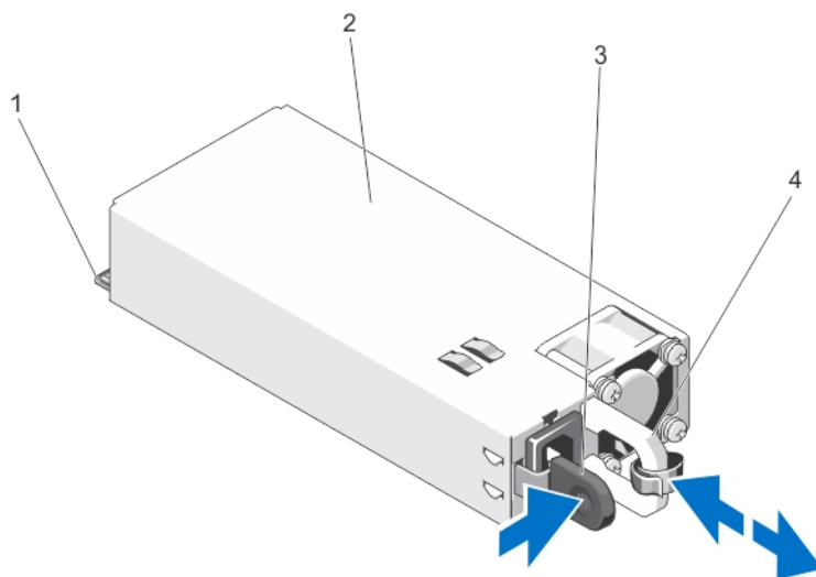
図 37. AC 電源装置の取り外しと取り付け
