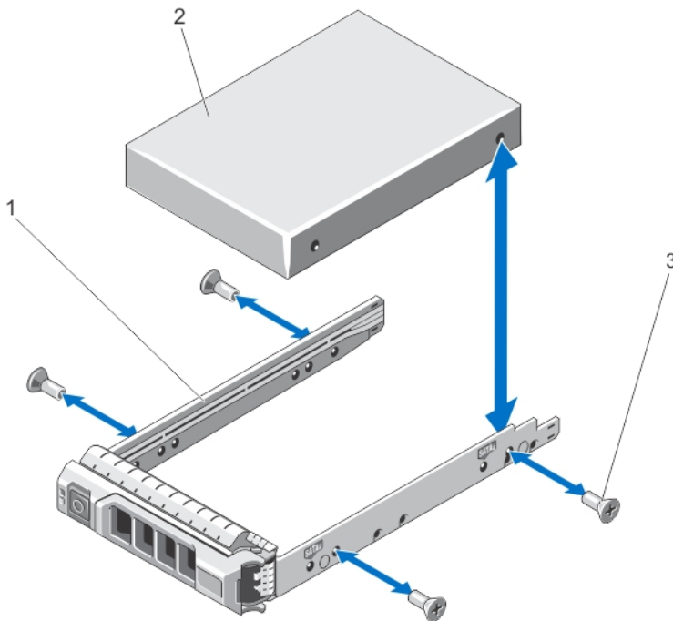
図 17. ハードドライブキャリアへのハードドライブの取り付けと取り外し
