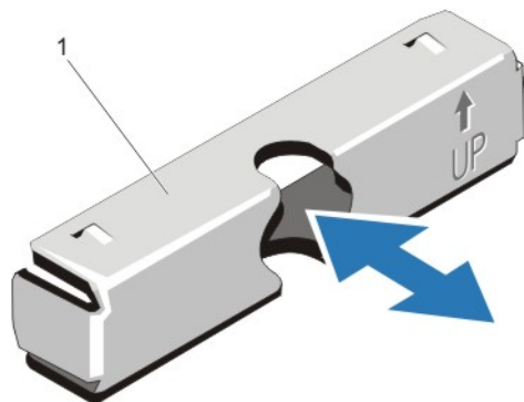
図 14. 2.5 インチハードドライブダミー（背面）の取り外しと取り付け
