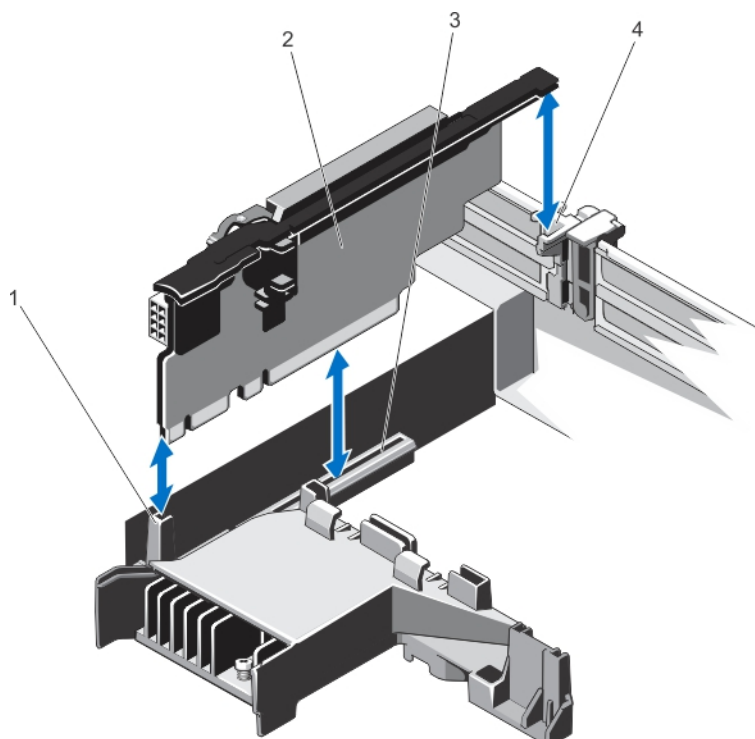
図 30. 拡張カードライザー 3 の取り外しと取り付け
